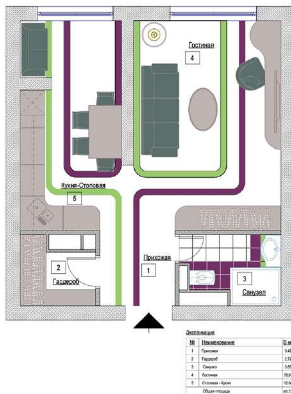
План квартиры с расстановкой мебели.
